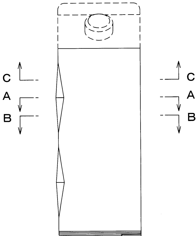
【正面図】
